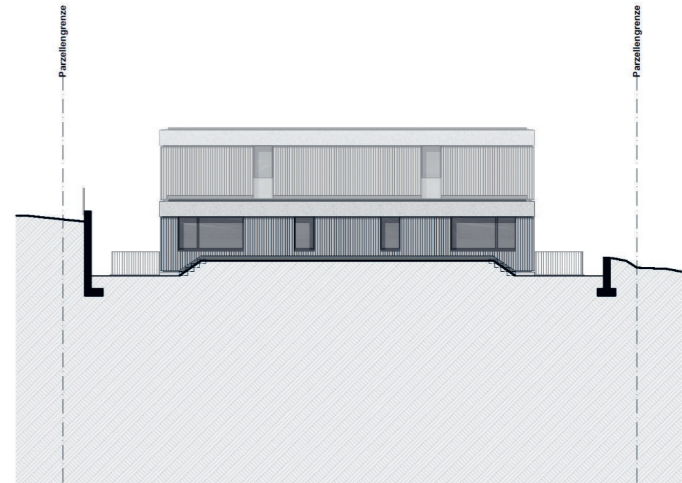
OSTFASSADE
