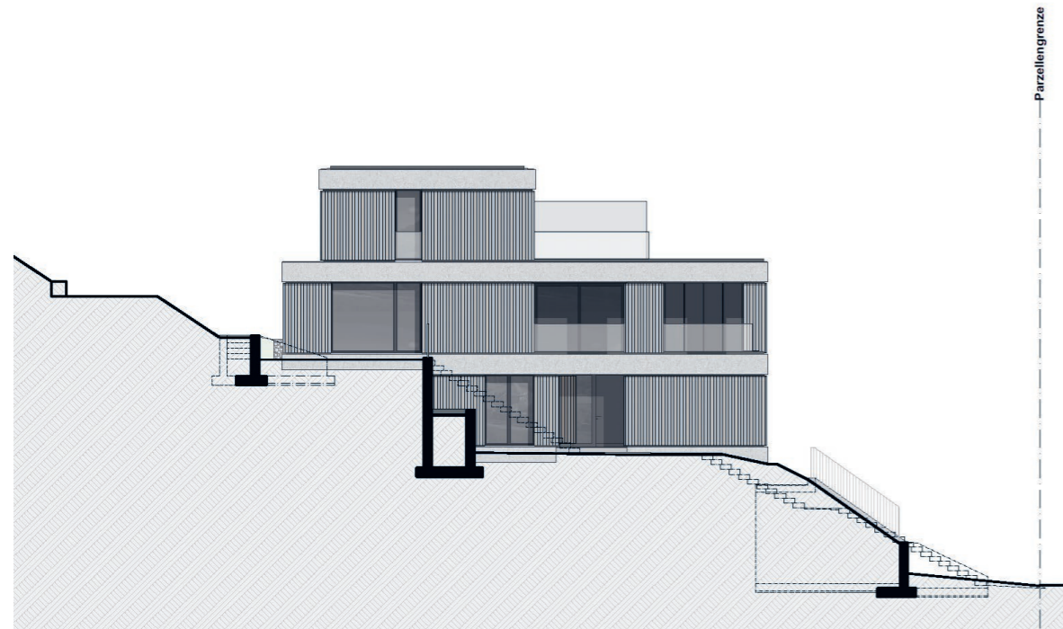
NORDFASSADE
